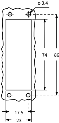
バルクヘッドハウジング用パネルカットアウト
