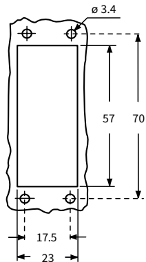
バルクヘッドハウジング用パネルカットアウト
